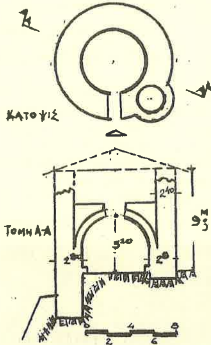
Κάτοψη και τομή του πύργου.
